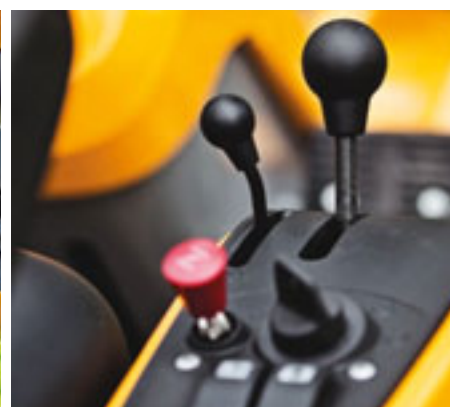
Páka hydraulického zvedání předních přídavných zařízení má čtyři polohy.
